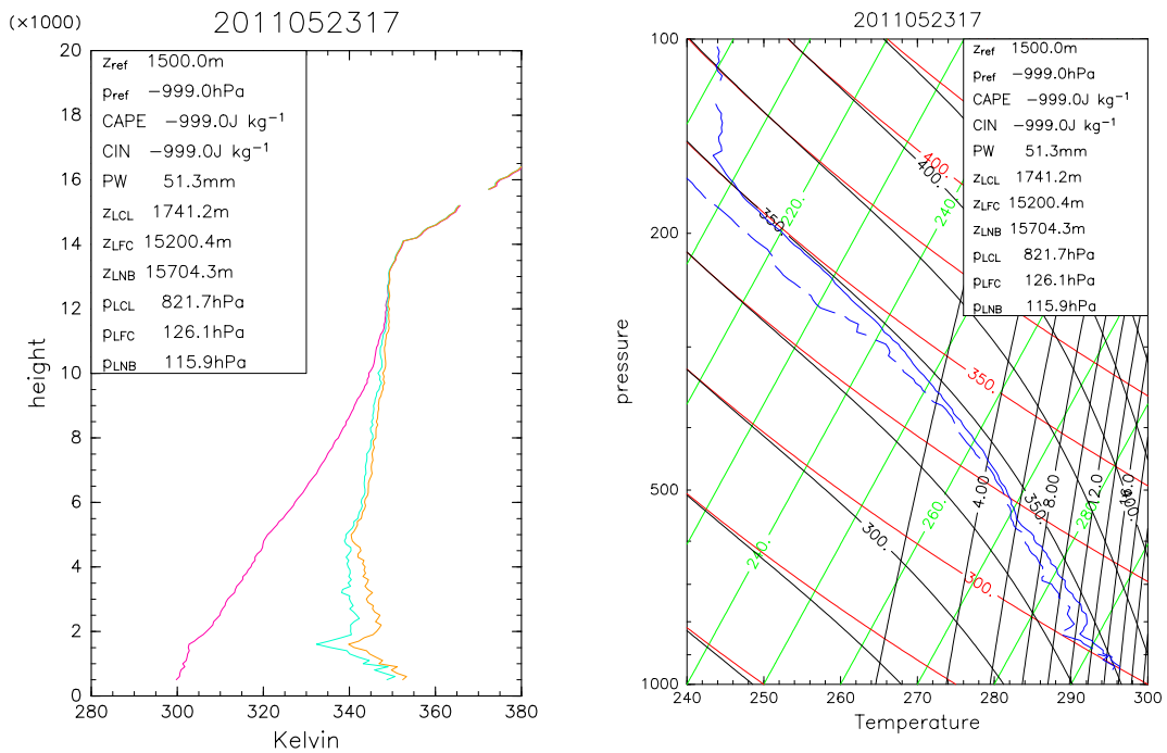
図 4.31: sound_1d で可視化されるサウンディングプロファイル (Skew-T 版). 図 4.32: sound_1d で可視化されるサウンディングプロファイル (エマグラム版).
