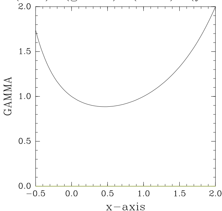
図 4.9: ガンマ関数.
