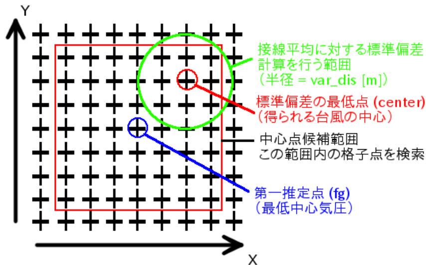
図 5.12: Braun 法の概念図 1. 第一推定点を中心に search_dis の長さの正方形領域 (赤線) 内に存在する格子点全てが中心点候補となる. この中心点候補の全てについて, 図 5.13 の方法で接線平均偏差を計算する (上図では緑線の範囲がそれに相当する).
