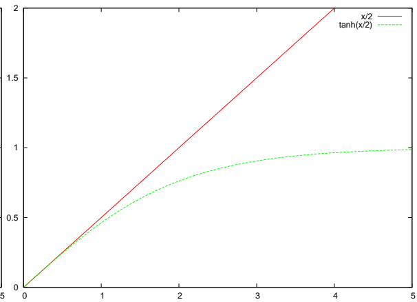
図 3.2: k/2 , \tanh(k/2) の関数形
